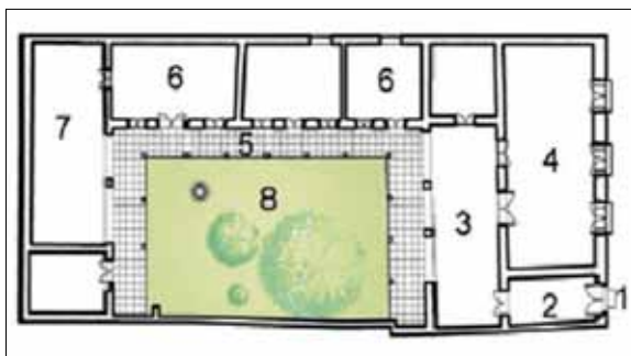
Иллюстрация 9. Жилой дом малого размера: 1 — вход; 2 — крыльцо; 3 — фойе; 4 — большой зал; 5 — коридор; 6 — спальня; 7 — столовая и кухня
