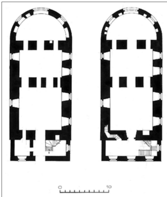
Иллюстрация 2. Чердынь. Иоанно-Богословская церковь. Постажные планы. Обмеры А. Б. Караева, Ю. Н. Потапова, А. В. Юдкина. 1973 г.
